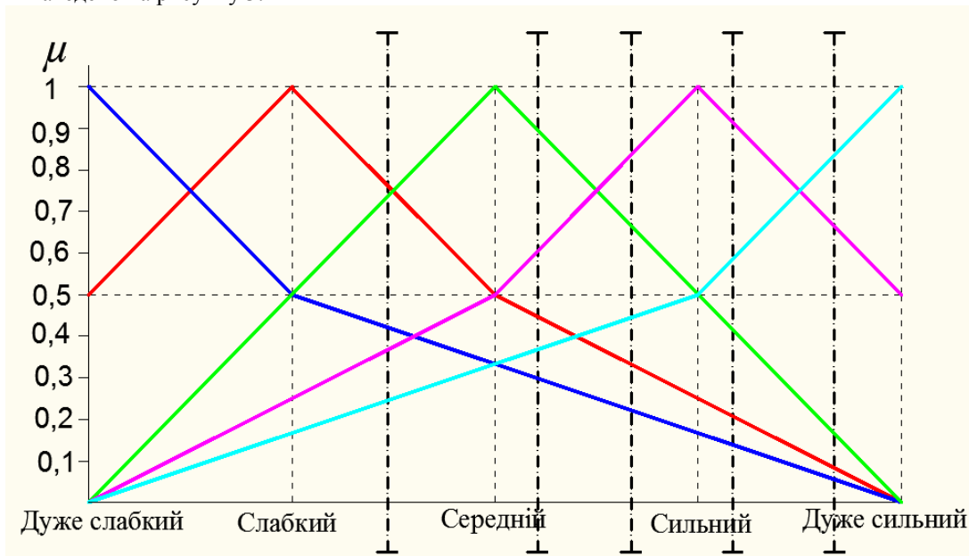
Рисунок 3 — Функції приналежності лінгвістичних оцінок ступеню впливу на енергоспоживання обсягу виробництва аміаку
