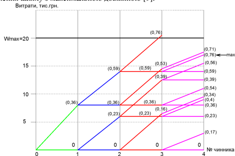
Рисунок 4 — Мережа, що ілюструє поетапне вирішення задачі про ранець.
