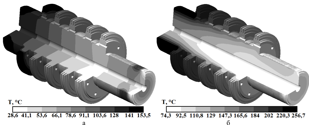
Рисунок 4 – Тепловий стан ротора високого тиску при пуску з НС-1 в момент часу: а – 100 с; б – 6600 с
