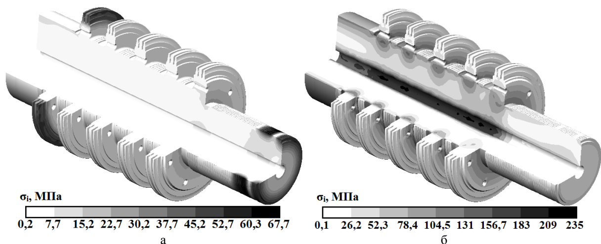
Рисунок 5 – Напружено-деформований стан PBT при пуску з нестиглого стану НС-1 в момент часу: а – 100 с; б – 6600 с
