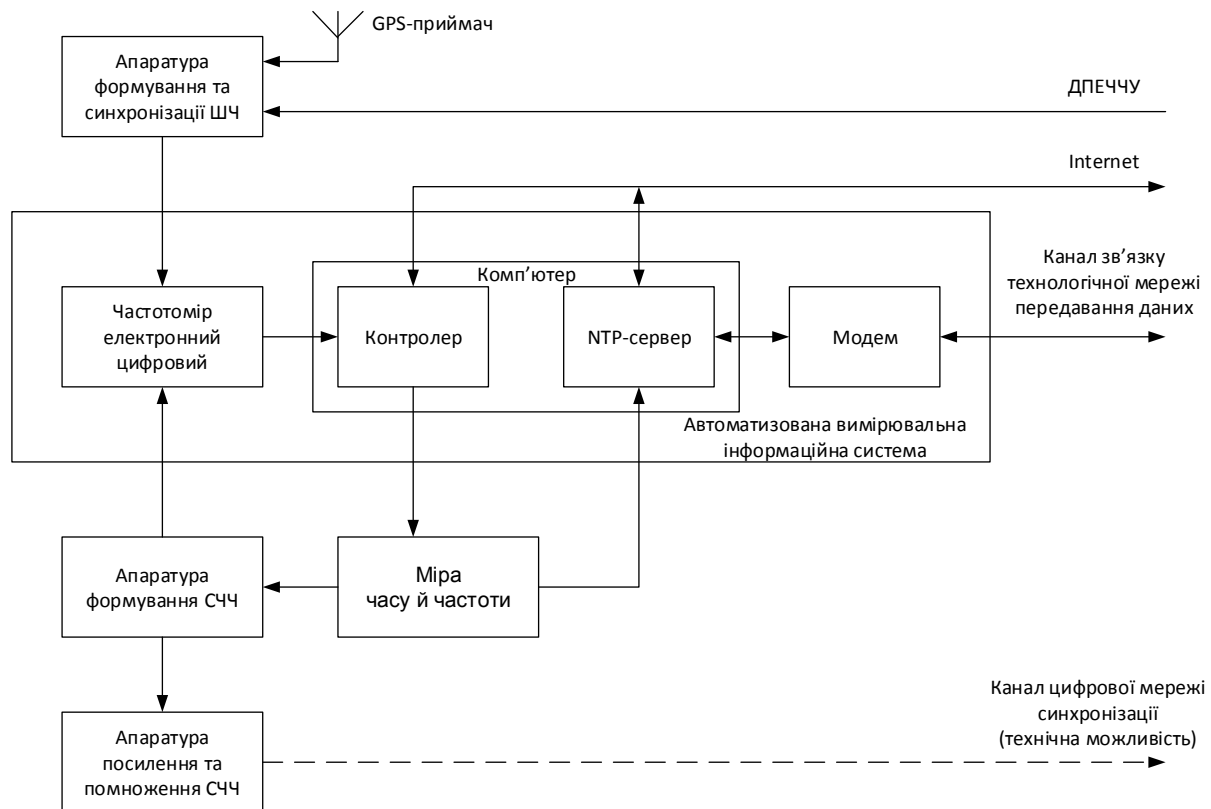
Рисунок 6 – Структурна схема пункту СТЧ лібералізованого ринку електричної енергії України
