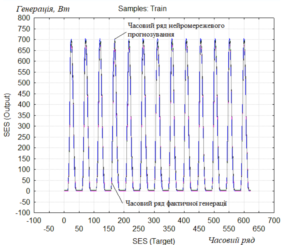
Рис. 4 – Результати нейронмережевого прогнозування генерації CEC
