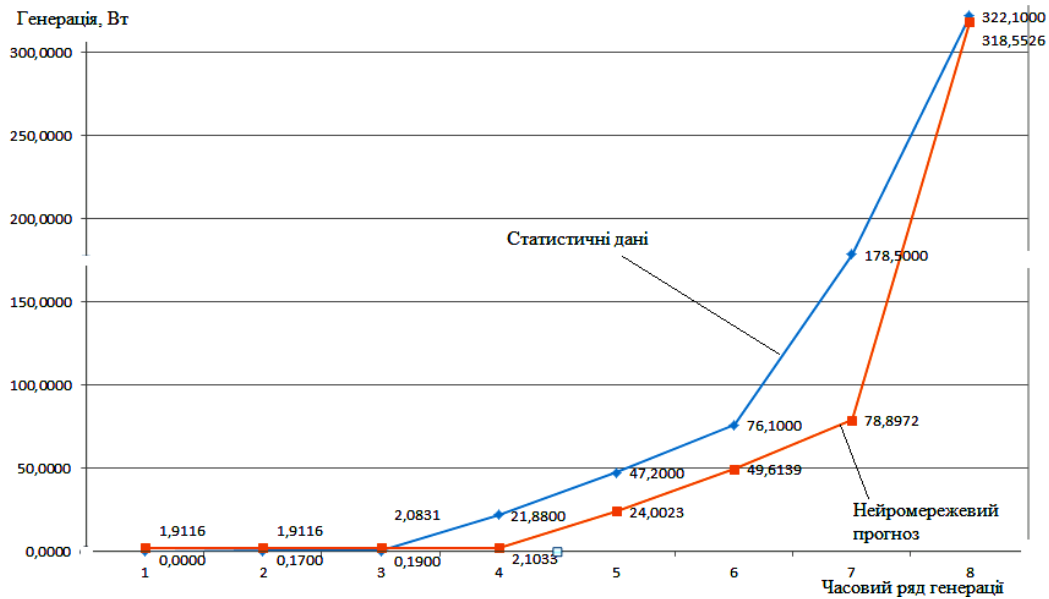
Рис. 5 – Приклад нейромережевого прогнозування генерації СЕС при її різких амплітудних змінах (багаточаровий перцептрон із 7 нейронами у прихованому шарі)
