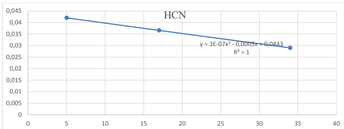
Рисунок 3 – Залежність кількості викидів від вологості спалюваної суміші для HCN
