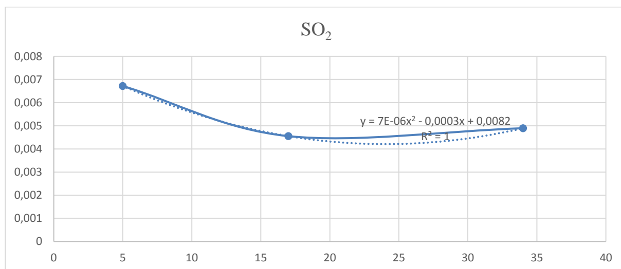
Рисунок 5 – Залежність кількості викидів від вологості спалюваної суміші для SO 2
