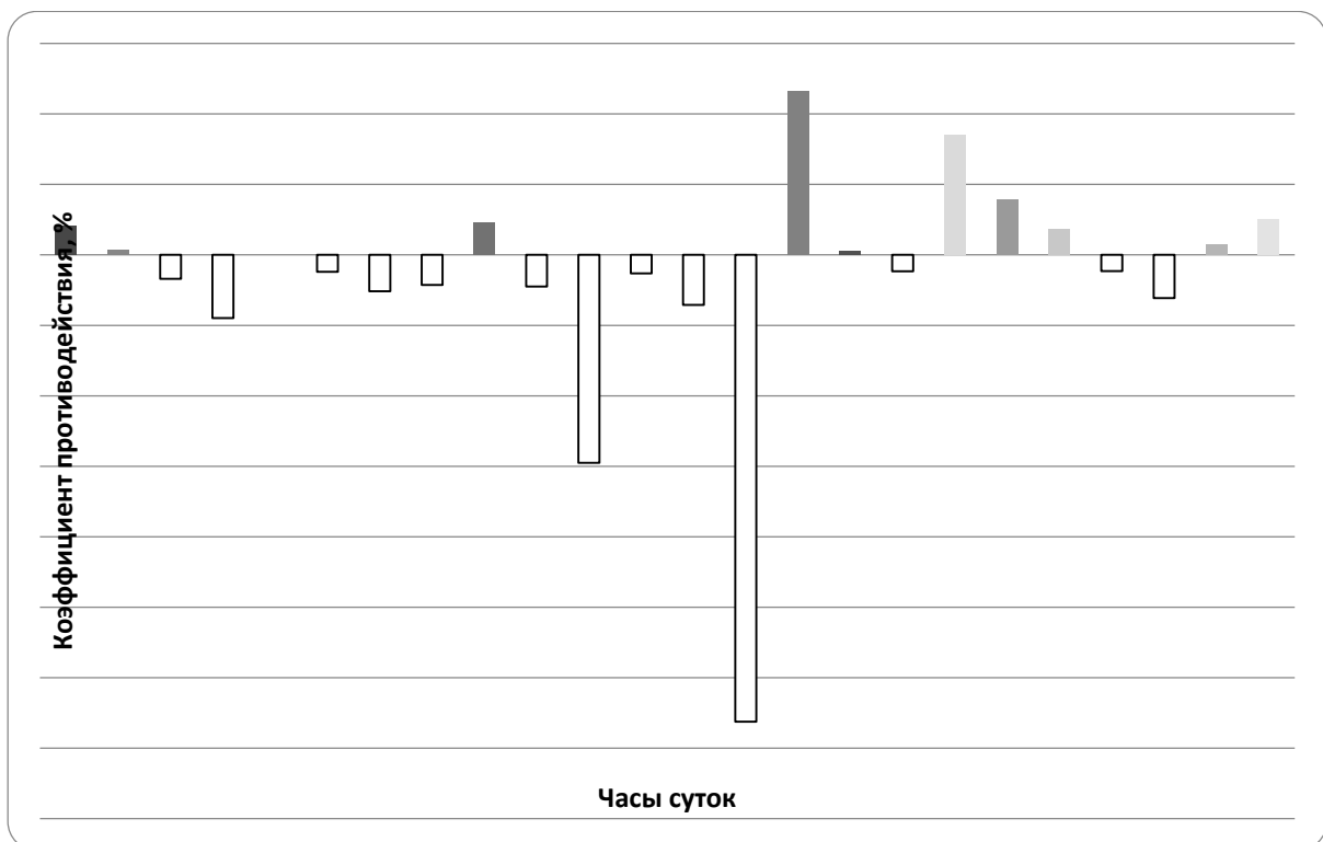
Рисунок 4 – Коеффіцієнти противодействія для часов суток, в которые изменение спроса на мощность «дифтарифных» потребителей оказывает негативное влияние на неравномерность графика нагрузки энергосистемы (зимний режимный день 21.12.2011 года).
