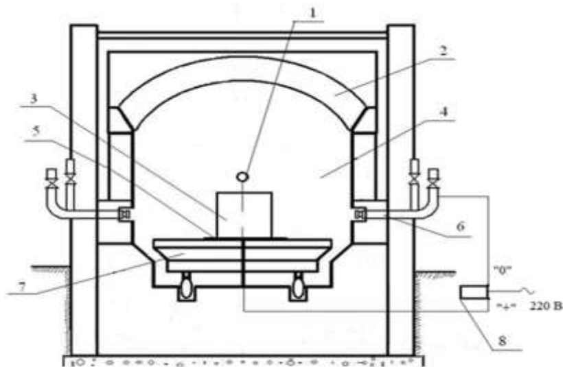
Рисунок1 – Схема застосування методу на камерній печі з підключеною електричною частиною: 1 – отвір для термопари, через який безконтактно вимірюється температура металу; 2 – склепіння; 3 – метал, що нагрівається; 4 – робочий простір; 5 – електропровідна пластина; 6 – пальник; 7 – викатний під; 8 – електрична частина
