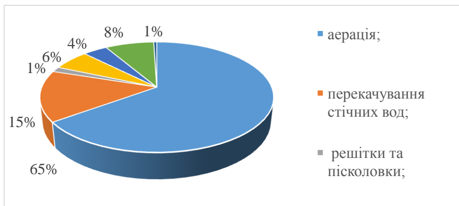
Рис. 1. Розподіл витрат електроенергії на каналізаційних очисних спорудах [3]
