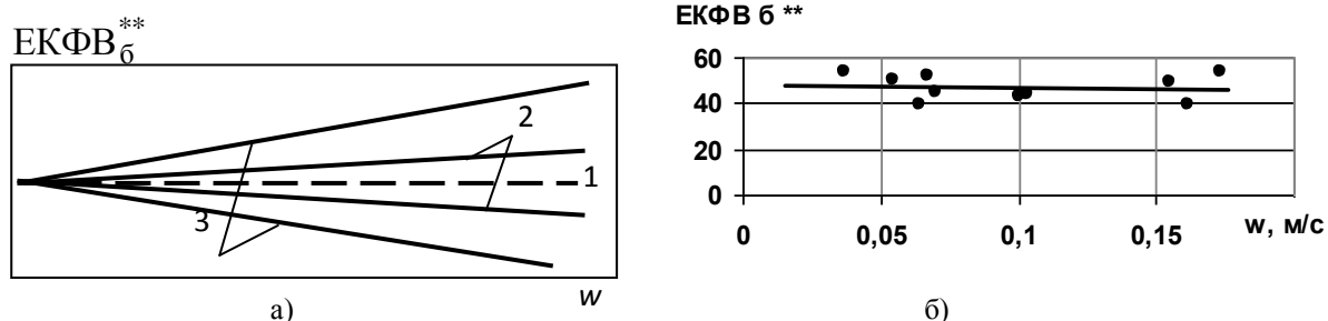
Рис. 1 Залежності \text{ЕКФВ}_{\bar{6}}^{**}(w) для різного класу рідин, які поводять себе як ньютонівське та неньютонівське середовище: а) якісні характеристики для: 1 – ньютонівська суміш; 2 – неньютонівська, близька до ньютонівської; 3 – неньютонівська; б) експериментальні точки, цукровий розчин концентрація 50%, \bar{t} = 40 \dots 45^\circ \text{C} (рідина з умовно невизначеними теплофізичними властивостями)
