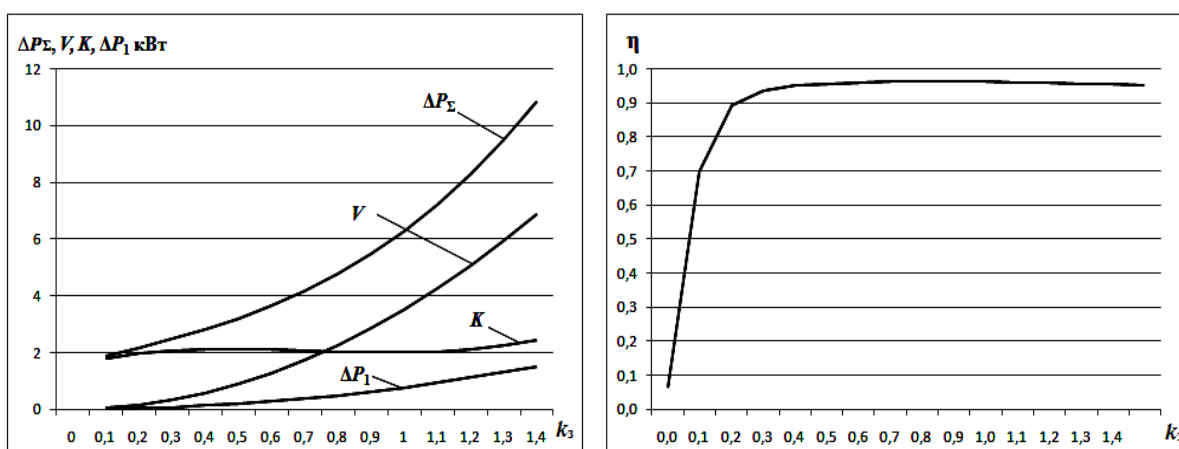
Рис. 4 Залежності параметрів процесу енерговикористання АД ( \Delta P_{\Sigma} , V , K , \Delta P_1 , \eta ) від коефіцієнта завантаження
