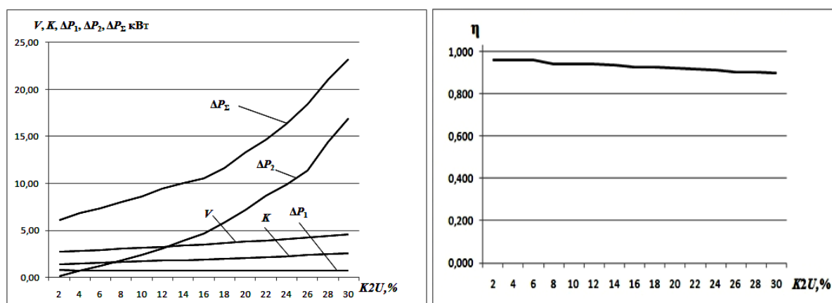
Рис. 8 Залежності параметрів АД ( \Delta P_2 , I , K , \Delta P_1 , \eta ) від несиметрії напруги
