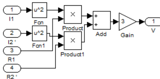
Рис. 3 Модель діагностування змінних втрат АД
