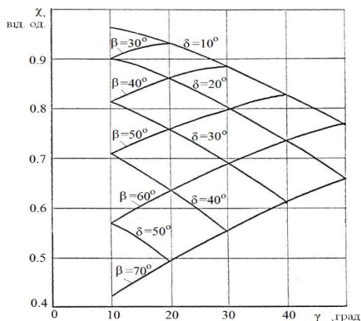
Рис. 2. Залежності коефіцієнта відносної потужності ВД від кутів параметрів і способів керування
