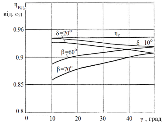
Рис. 4. Залежності ККД ВД від кутів параметрів і способів керування
