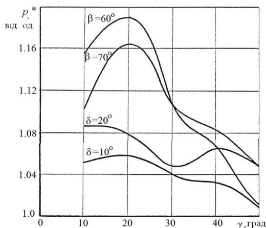
Рис. 2. Залежності коефіцієнта відносної потужності ВД від кутів параметрів і способів керування
