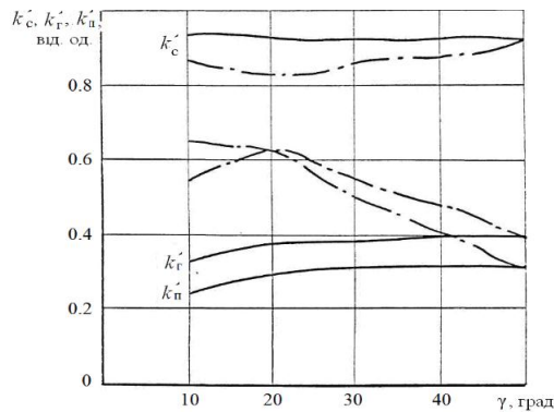
Рис. 1. Криві залежності коефіцієнтів k'_c, k'_r, k'_II від кута комутації: — \beta_{\min}=f(\gamma) за умови \delta=10^\circ ; - - \beta=60^\circ=\text{const}
