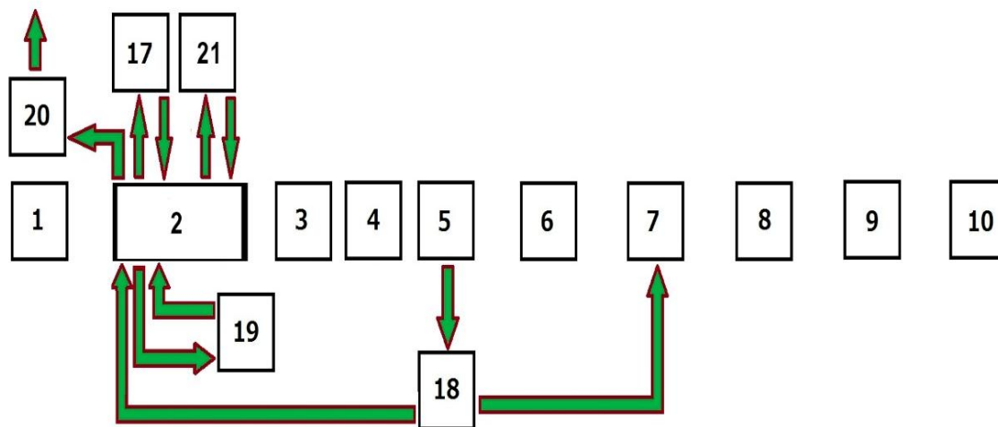
Рисунок. Схема лінії травлення друкованих плат з відведенням на регенерацію: 1 – модуль завантаження; 2 – травильний модуль; 3 – модуль освітлення; 4 – оглядовий модуль; 5 – третій модуль каскадного промивання; 6 – другий модуль каскадного промивання; 7 – перший модуль каскадного промивання; 8 – модуль гарячого сушіння; 9 – модуль холодного сушіння; 10 – модуль вивантаження; 17 – регенератор травильного розчину; 18 – регенератор промивних вод; 19 – фільтраційна установка; 20 – очисні споруди підприємства; 21 – установка нанесення покриттів (за необхідності).
